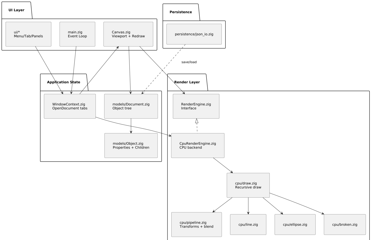
Figure 1: Компонентная архитектура Zivro
